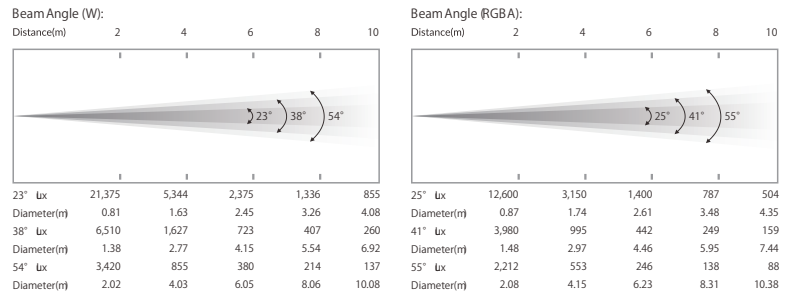
照度図
