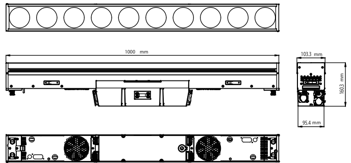
寸法図(mm)
