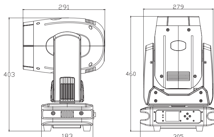
寸法図
