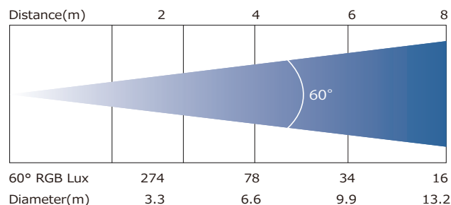
照度図
